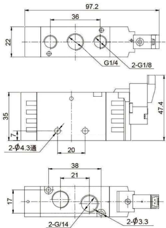
5V200M系列-2位单电控
