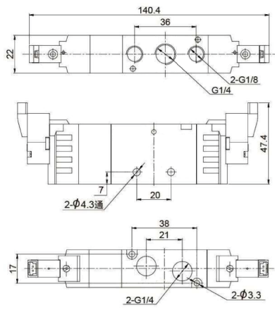
5V200M系列-3位双电控
