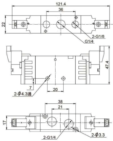
5V200M系列-2位双电控
